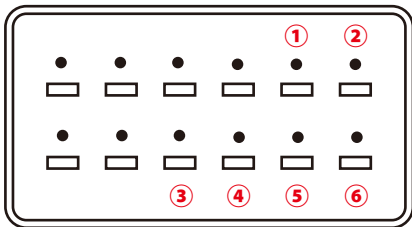
コネクタ正面図
